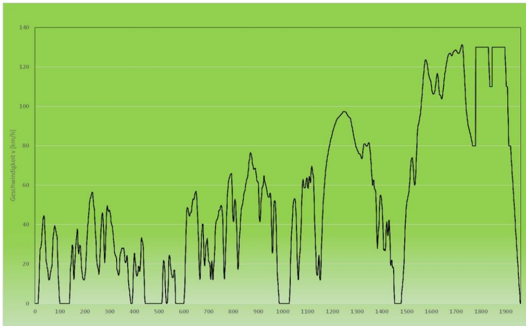
Abbildung 1: ADAC Elektrozyklus
